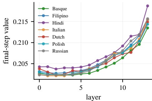
Hoyer( W_{\text{SwiGLU}} )
