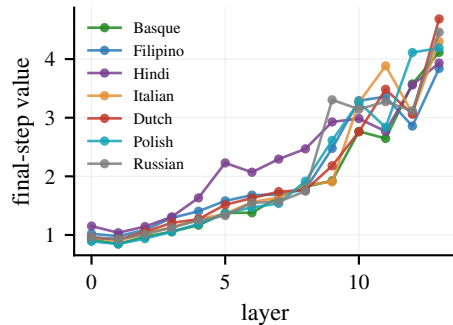
\|W_{OV}\|_F
