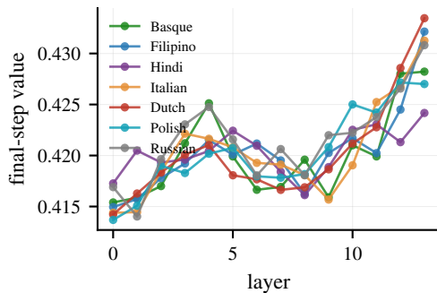
Hoyer( W_{\text{SwiGLU}} )
