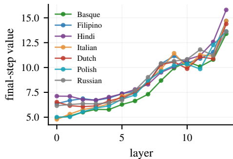
\|W_{OV}\|_F
